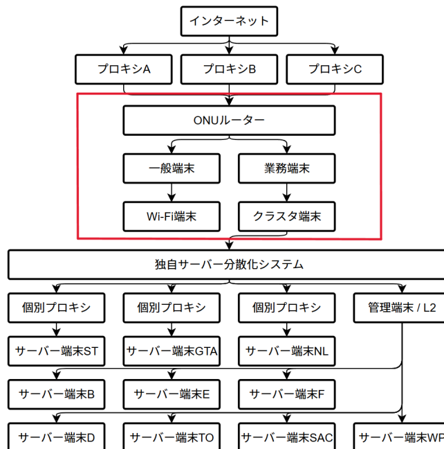
Figure 1: nyaisaba.com 横浜DC システム概要図(2026年06月)
